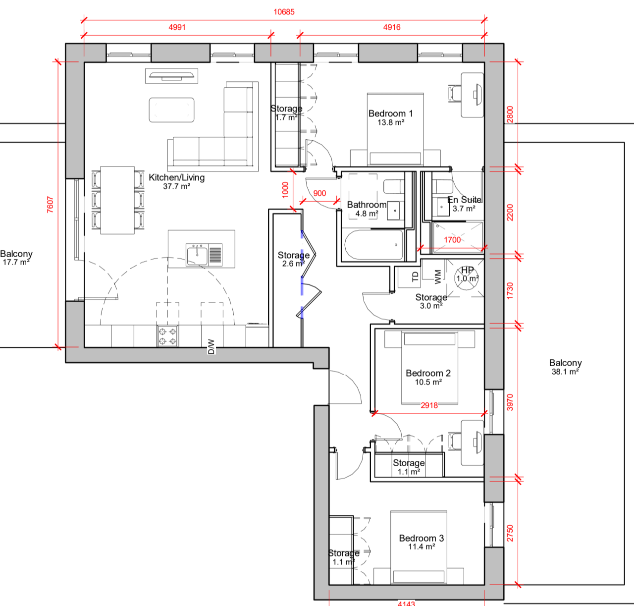
3 3 BED TYPE C 1 : 100
