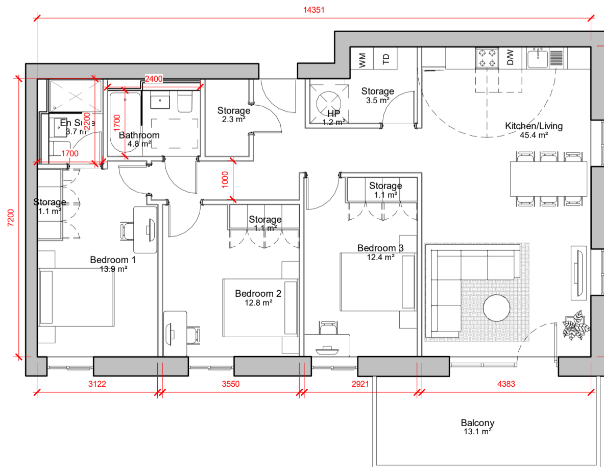
8 3 BED TYPE H 1 : 100
