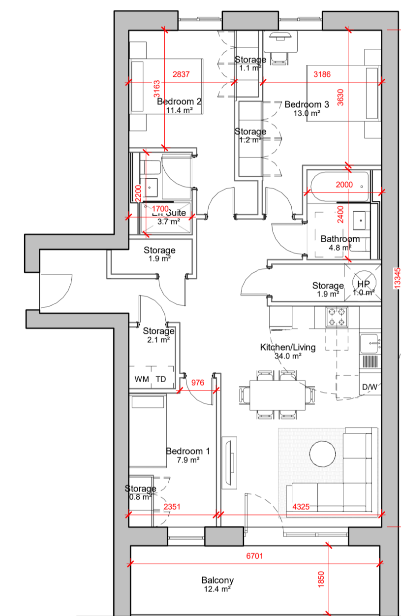
5 3 BED TYPE E 1 : 100
