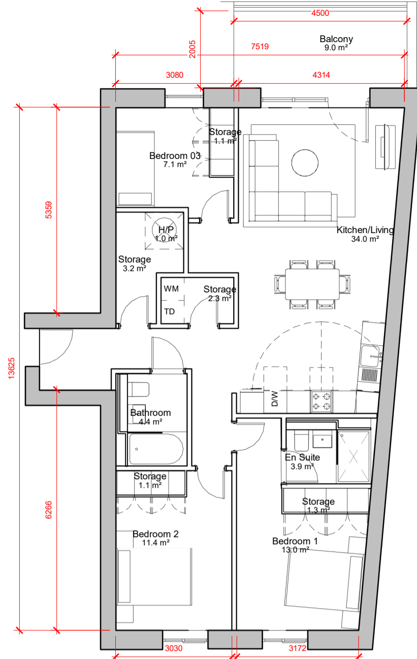
1 3 BED TYPE A 1 : 100
