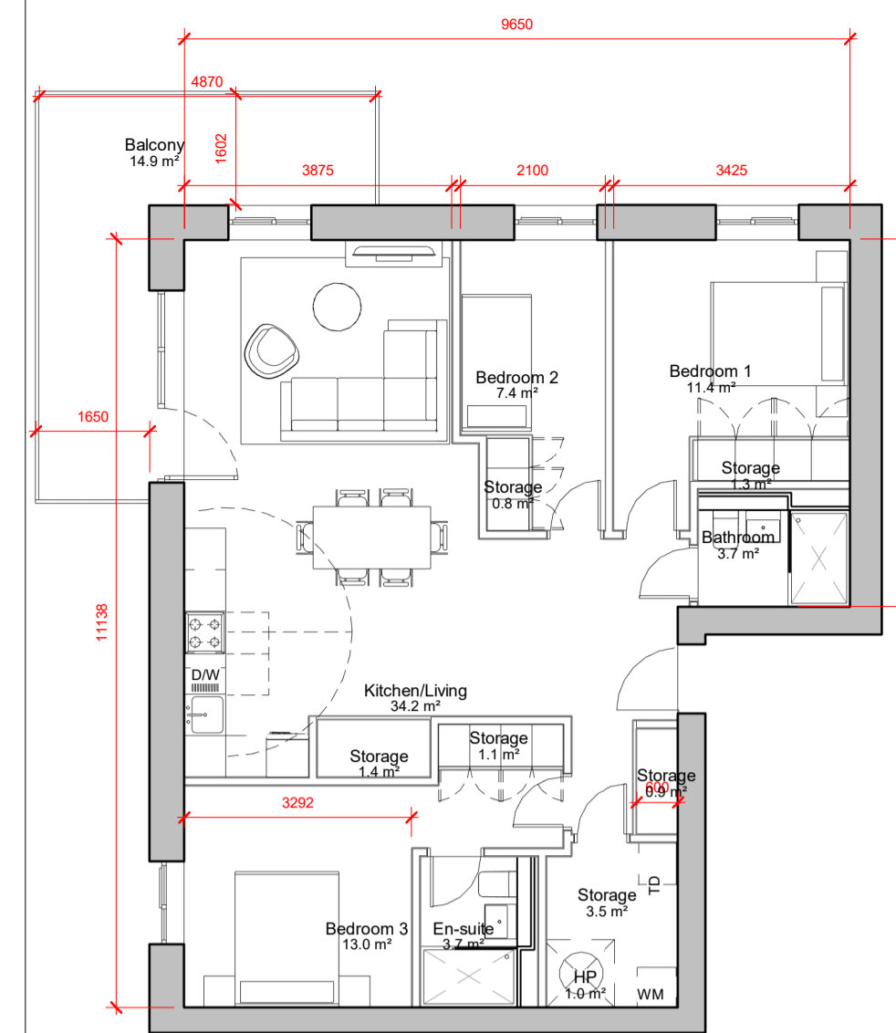
9 3 BED TYPE B2 1 : 100
