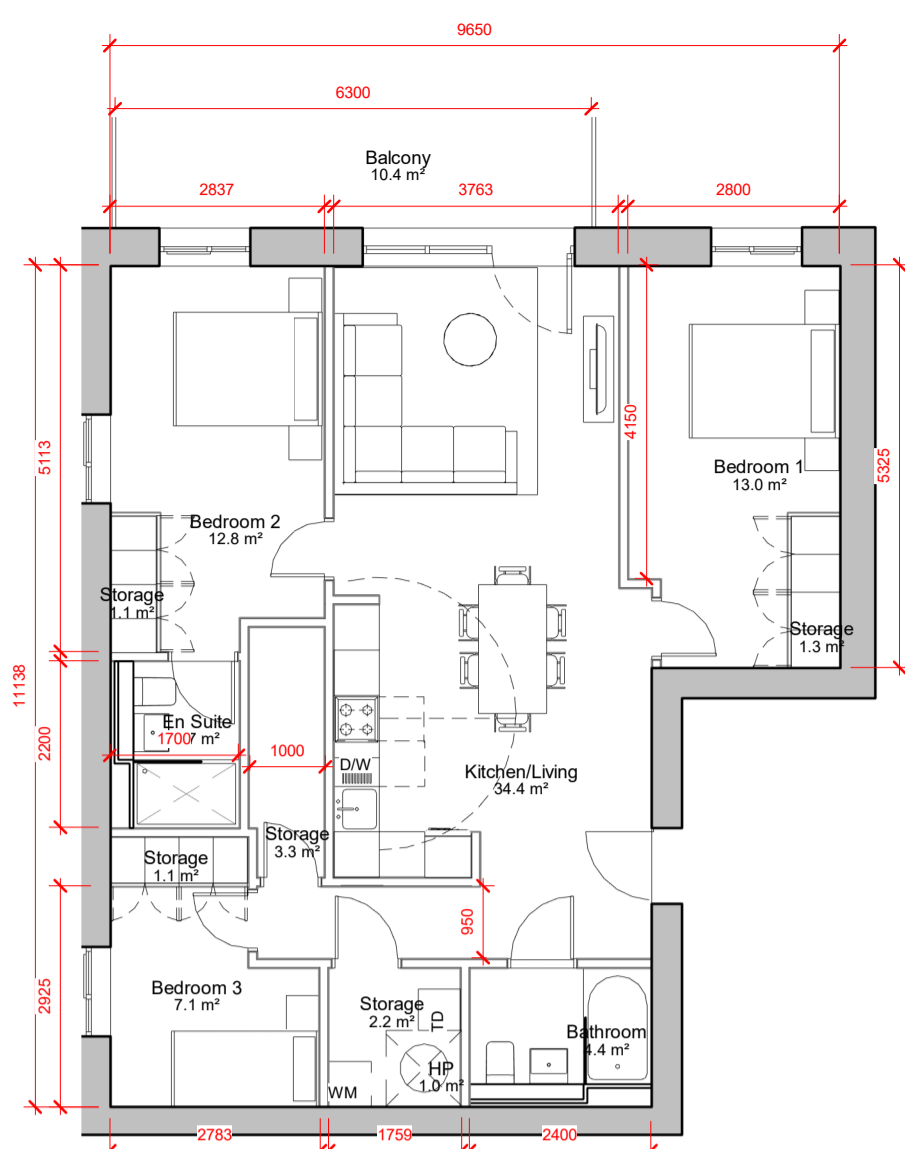
2 3 BED TYPE B 1 : 100
